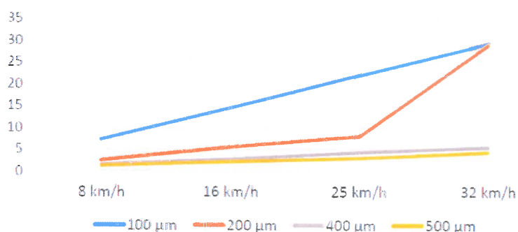
% de dérive en fonction de la vitesse du vent et de la taille des gouttelettes
