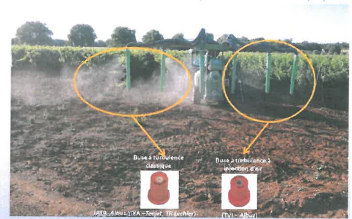
Comparaison de différentes buses sur un pulvérisateur viticole à jet porté
